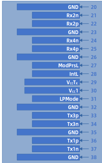
顶部直视图
